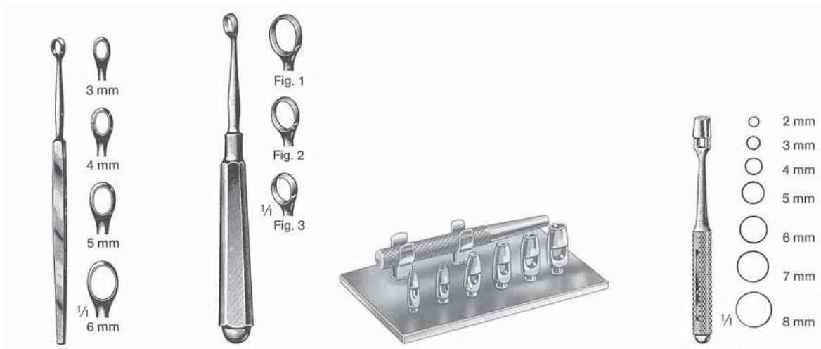
mm FOX 3 HI.128.03 4 HI.128.04 5 HI.128.05 6 HI.128.06
